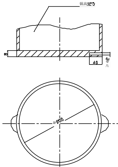
图 C. 2 试验用油锅
