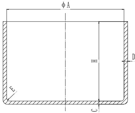
图 21 试验用锅筒图
