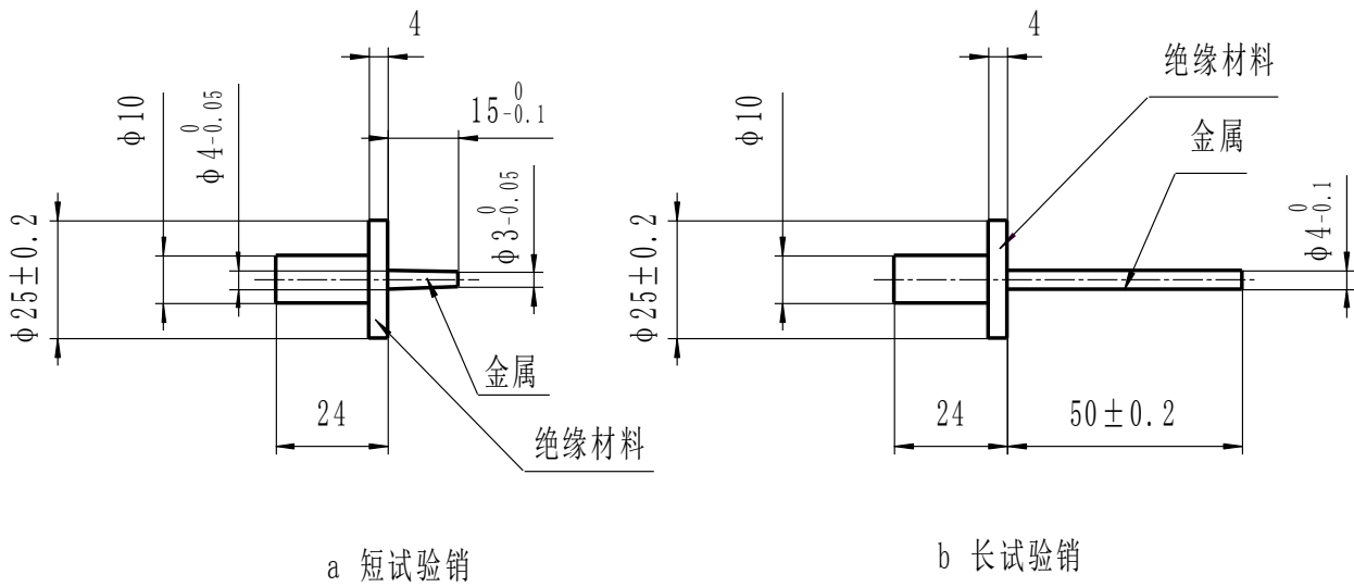
图3 试验销
