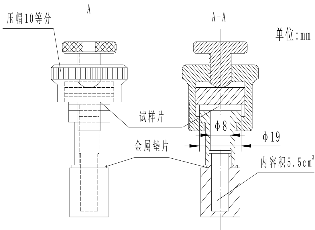
图 18 垫圈、垫片耐燃气试验装置
