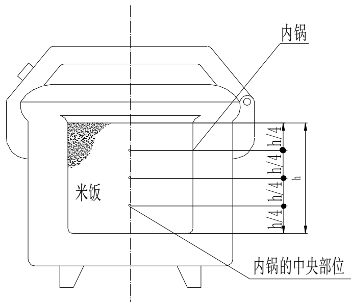
图 10 灶具与测温板的距离
