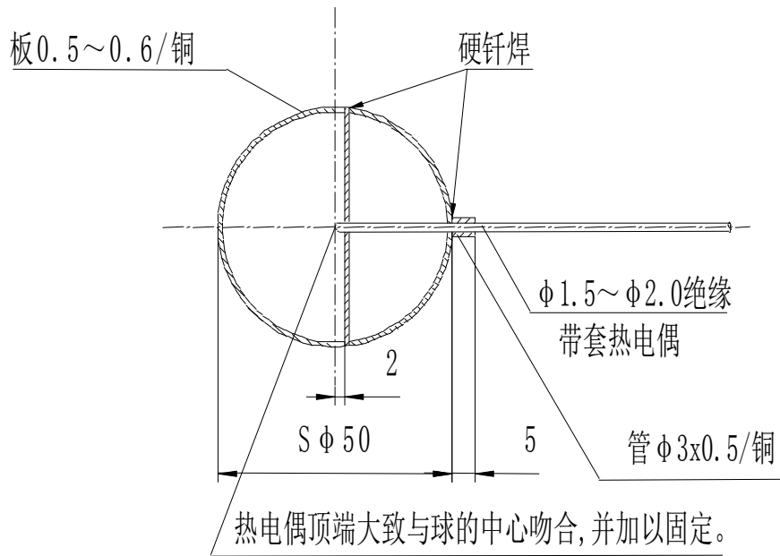
图 14 测定烤箱温度用热电偶
