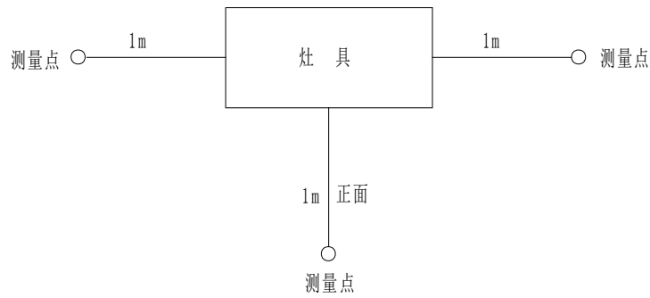
图 5 噪声测定示意图
