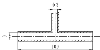
a) 试验装置连接图
